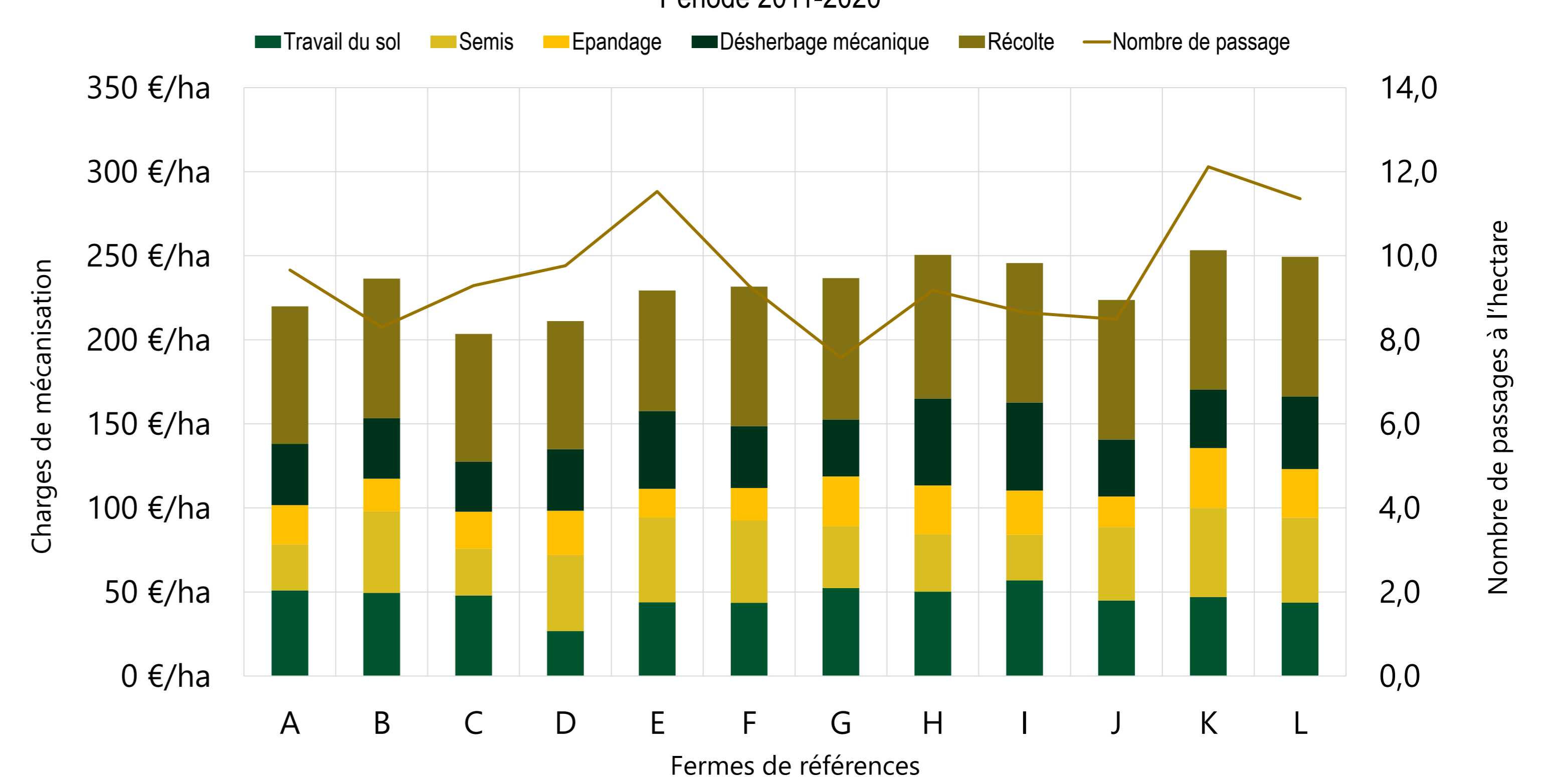
Charges de mécanisation par type d'intervention, par hectare et par exploitation Données réseau de fermes de références Période 2011-2020
