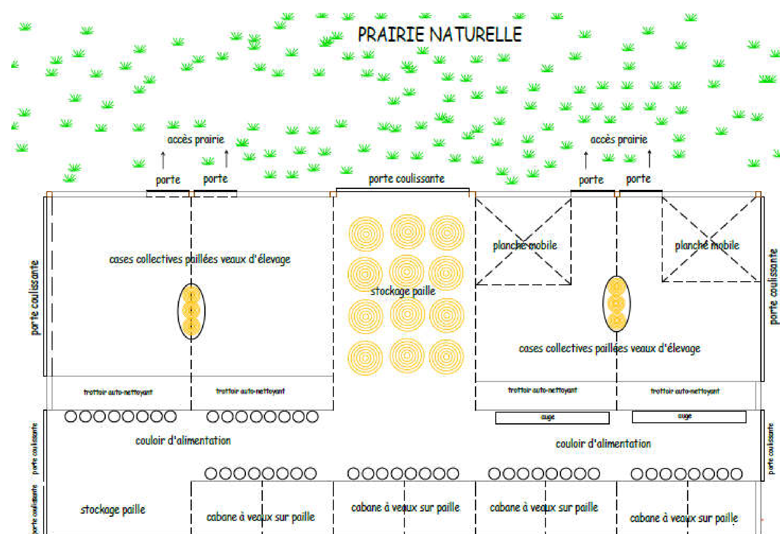
Exemple de plan d'aménagement d'une nurserie avec accès au pâturage
