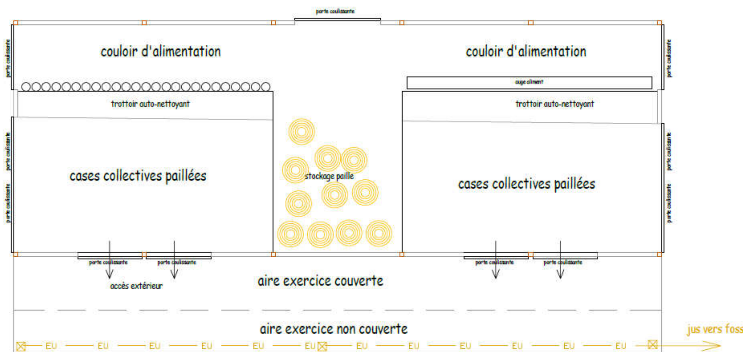
Exemple de plan d'aménagement d'une nurserie avec accès aire d'exercice
